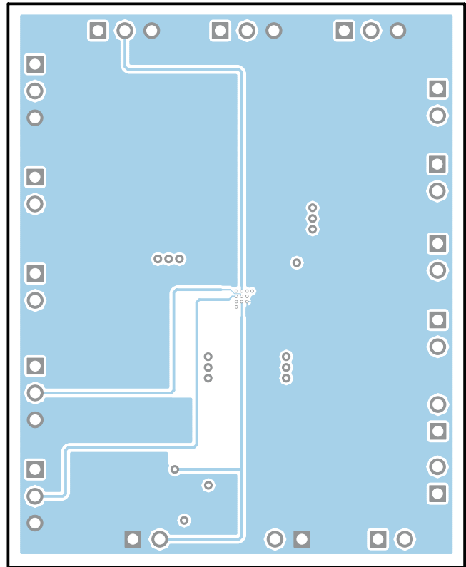
Figure 21. EVM Layer 2
